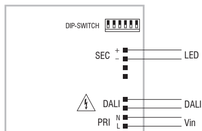
DALI diagram - Collegamento DALI
