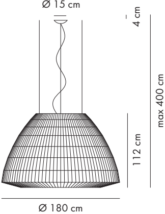
SPBEL180
