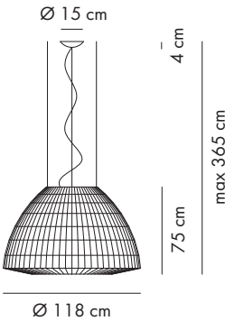
SPBEL118
