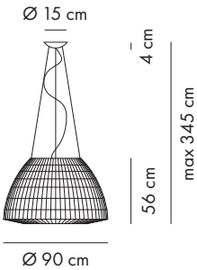
SPBEL180
